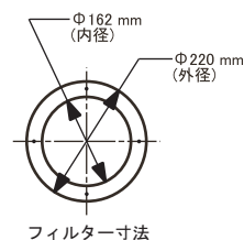
フィルター寸法
